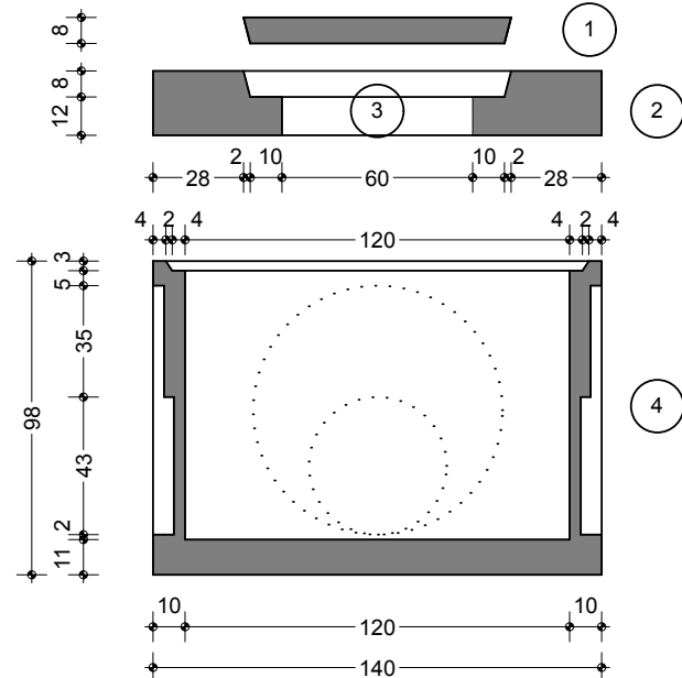
SEZIONE POZZETTO A-A SCALA 1:25
