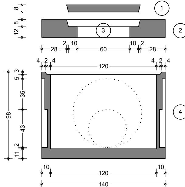
SEZIONE POZZETTO B-B SCALA 1:25
